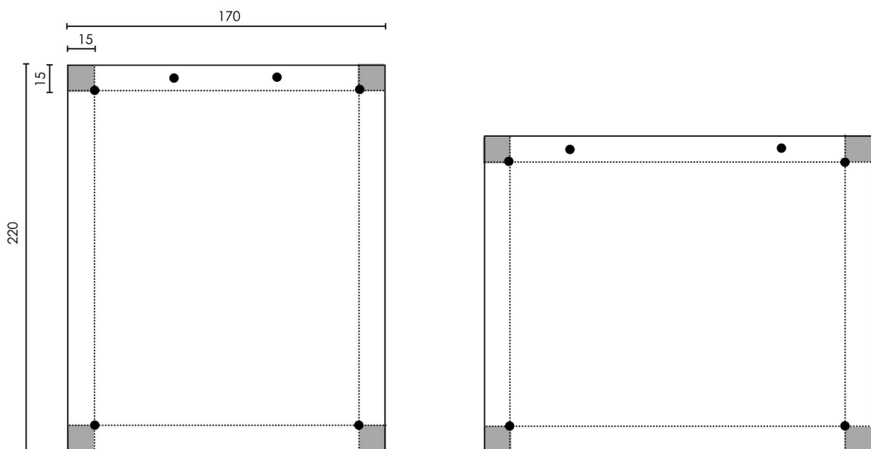
tekening 1: memobord: rechtop of liggend
